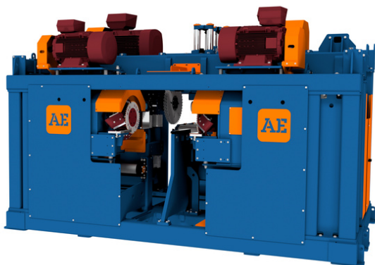
CENTRE DELIGNEUSE MODULAIRE CDM 225-250
